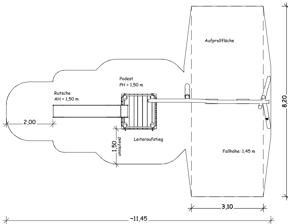
Draufsicht
